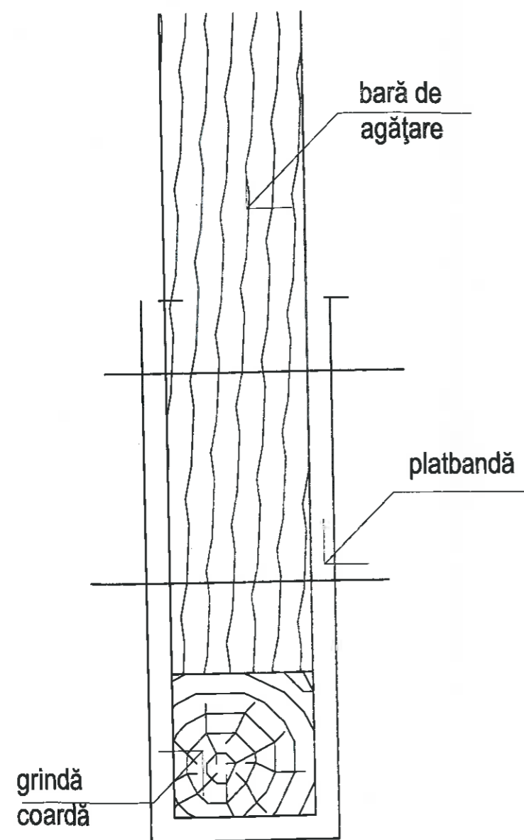
SECȚIUNE
