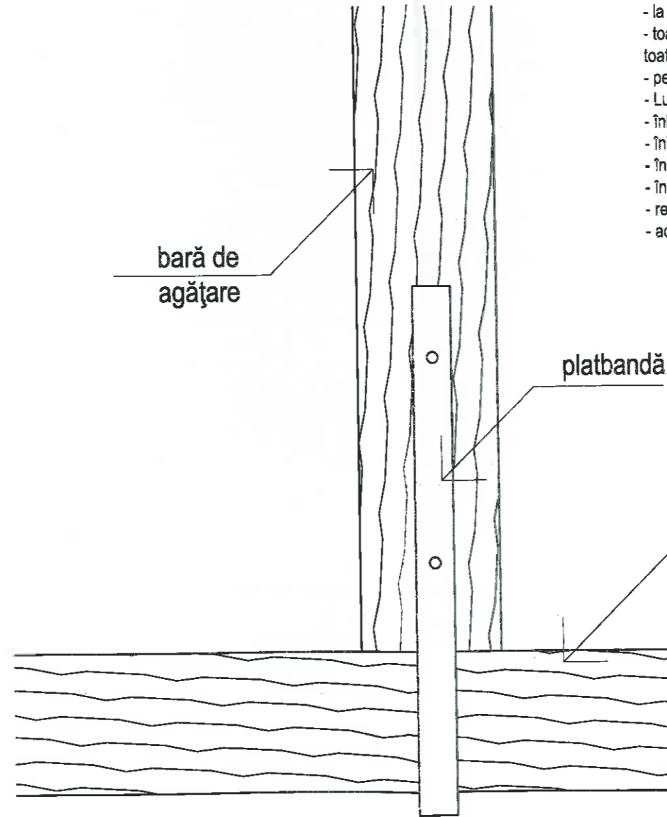
VEDERE LATERALĂ
