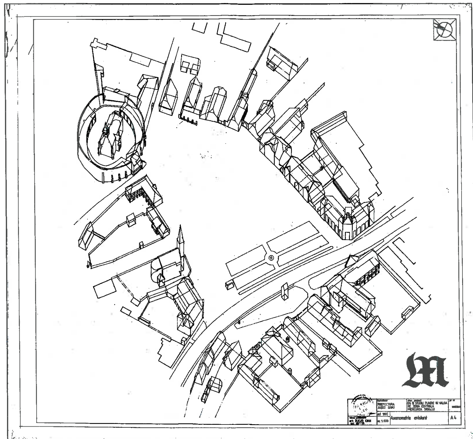
img. 7 Piața centrală - axonometrie situația existentă 1990
