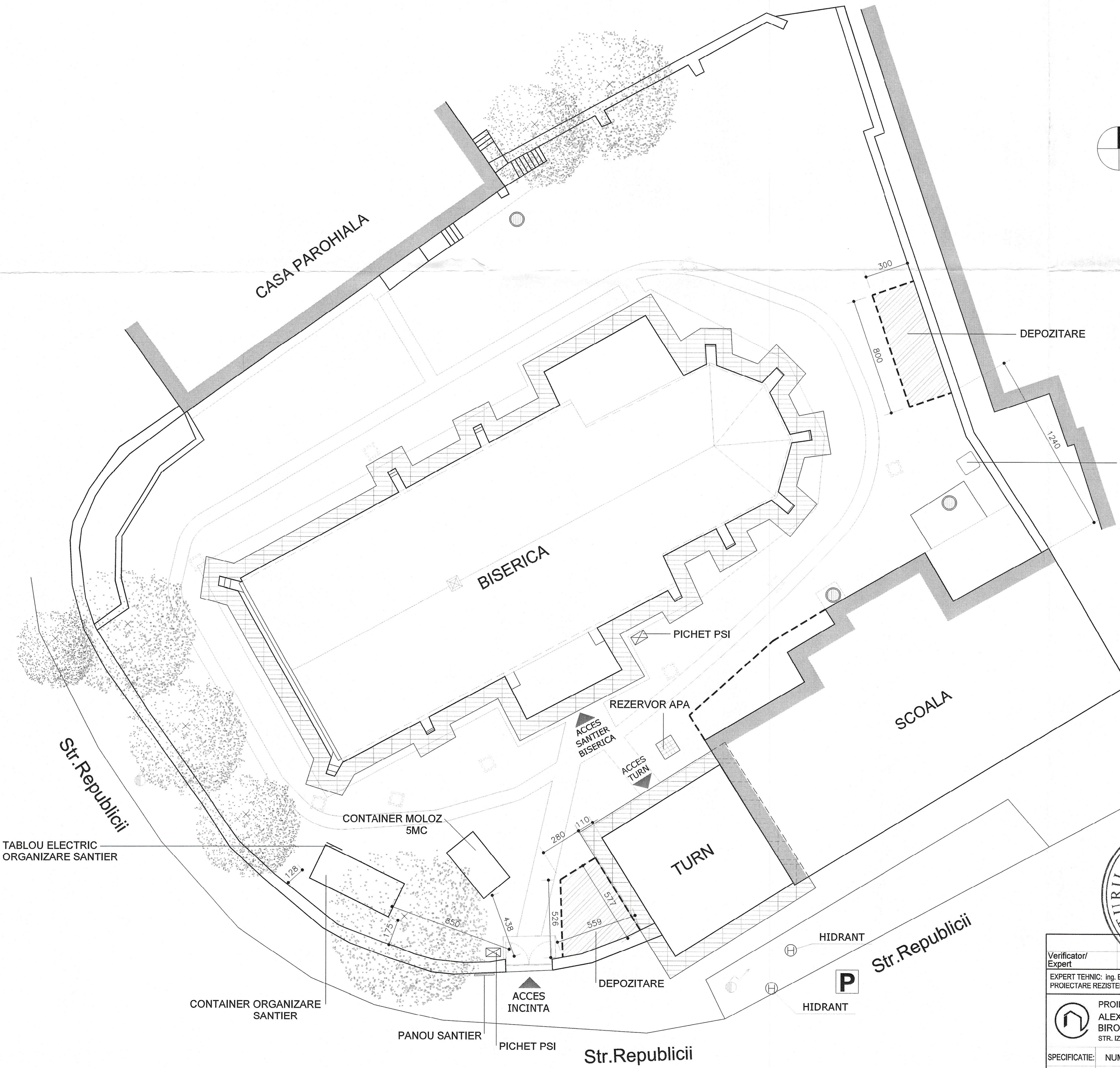
PLAN DE SITUATIE - PROPUNERE
