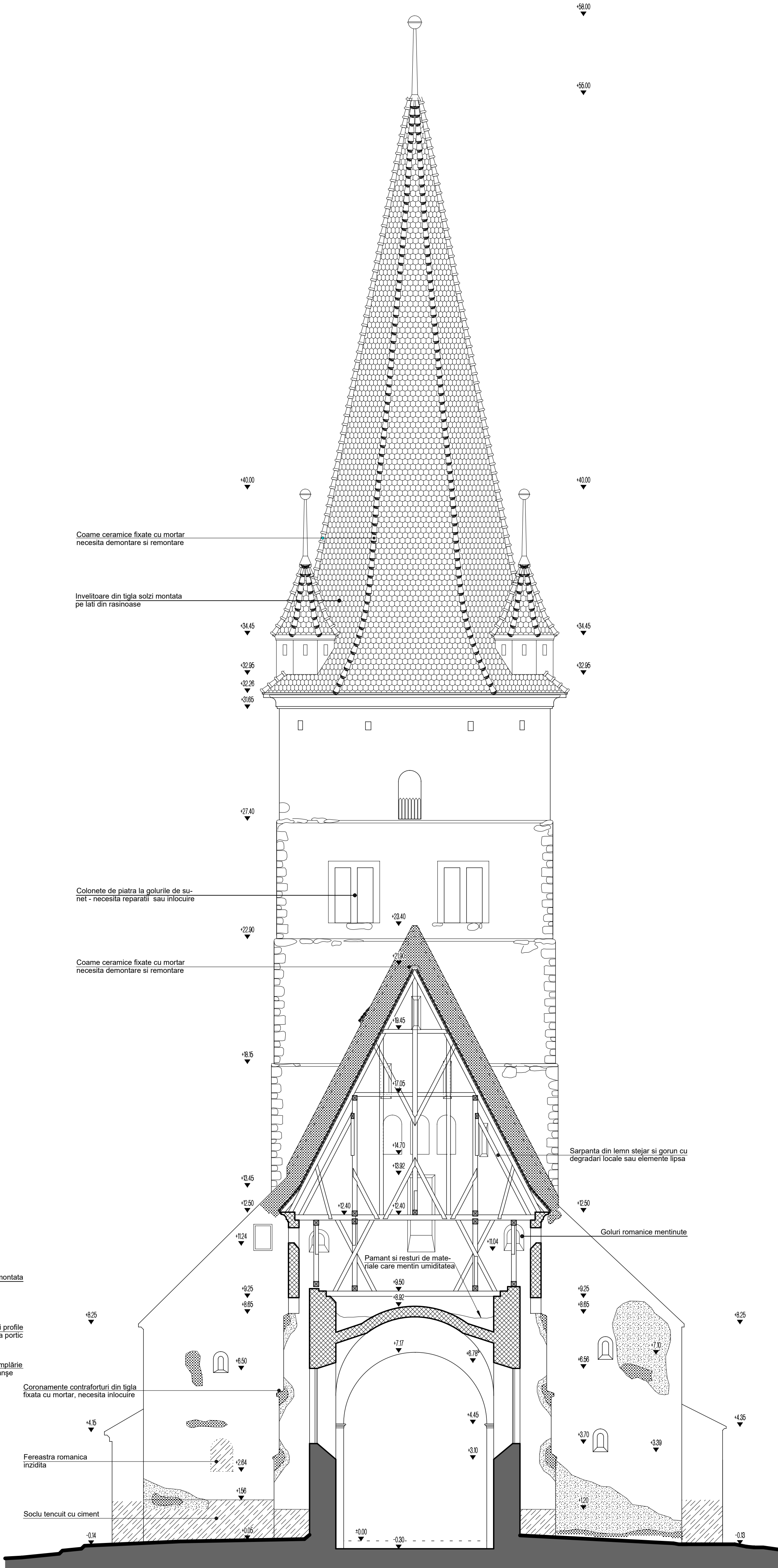
RELEVU BISERICA - SECTIUNE C-C scara 1:100
