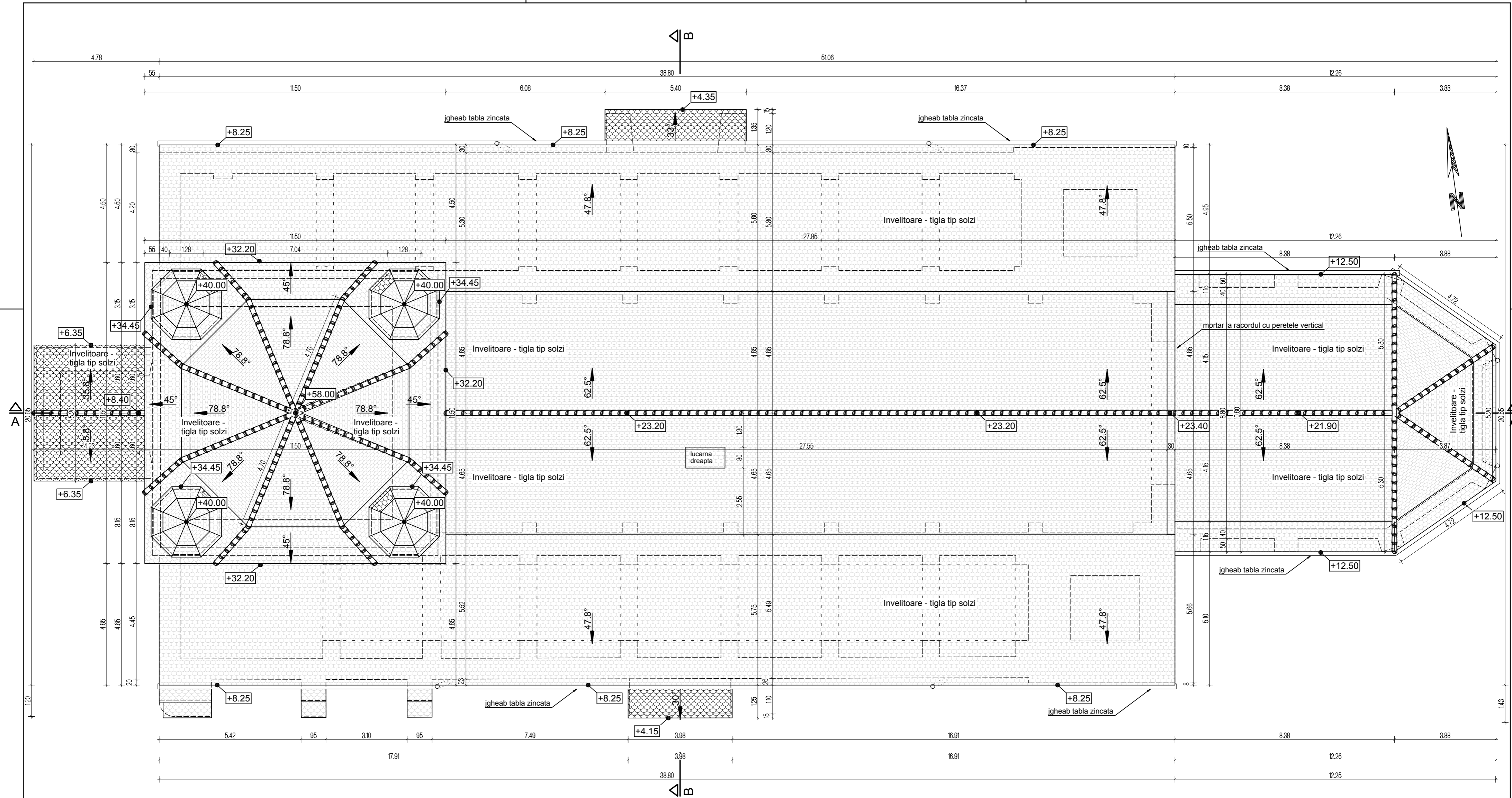
RELEVU BISERICA - PLAN EMPORE SI NIVEL 1 TURN (COTA +6.00) scara 1:100
