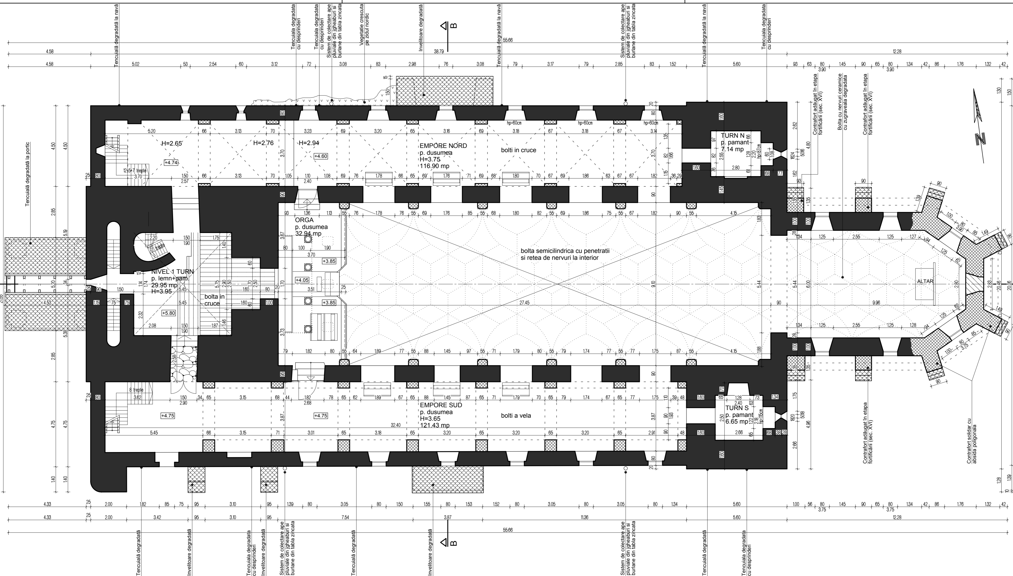
RELEVU BISERICA - PLAN EMPORE SI NIVEL 1 TURN (COTA +6.00) scara 1:100
