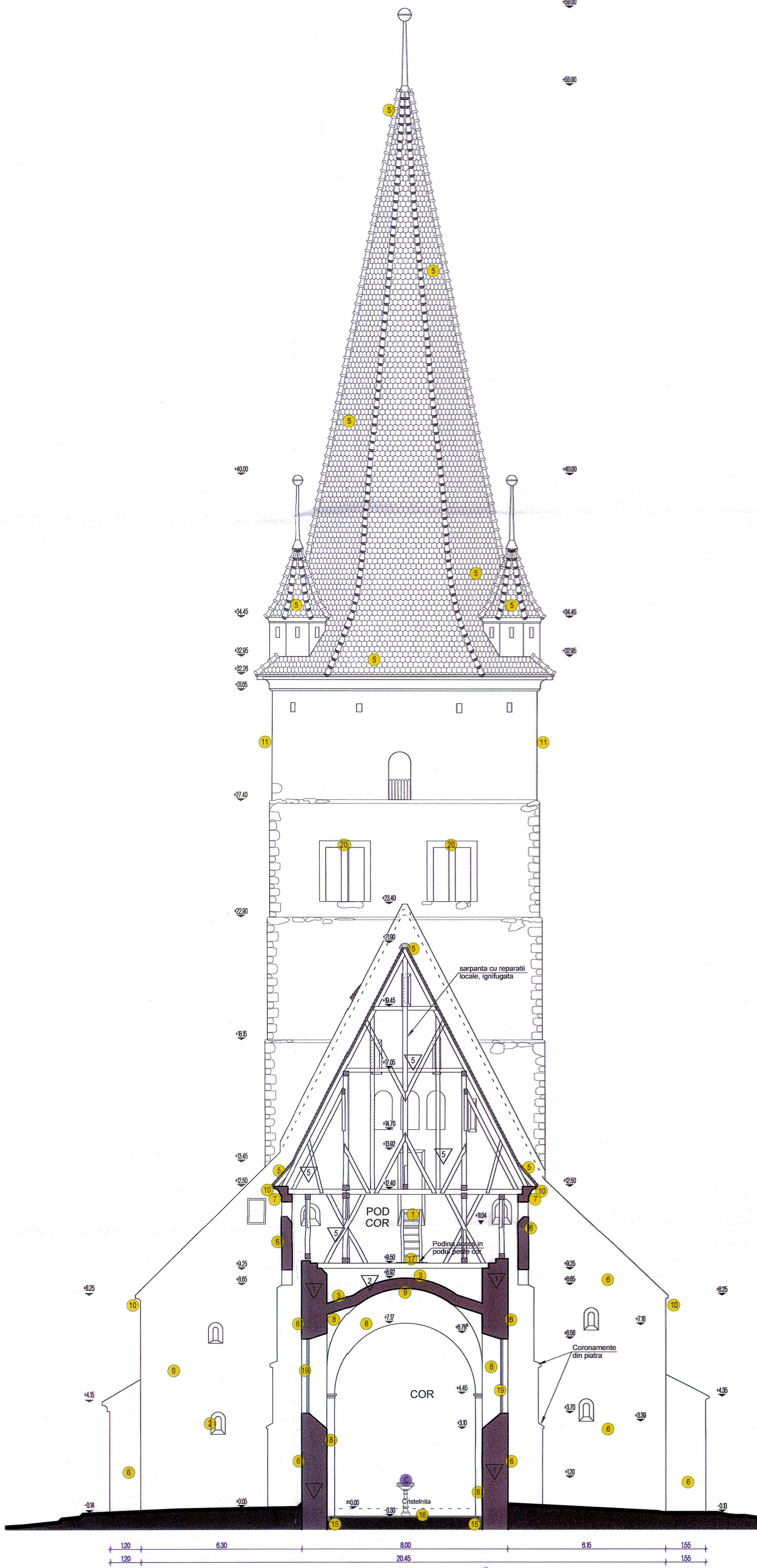
PROPUNERE BISERICA - SECTIUNE C-C scara 1:100
