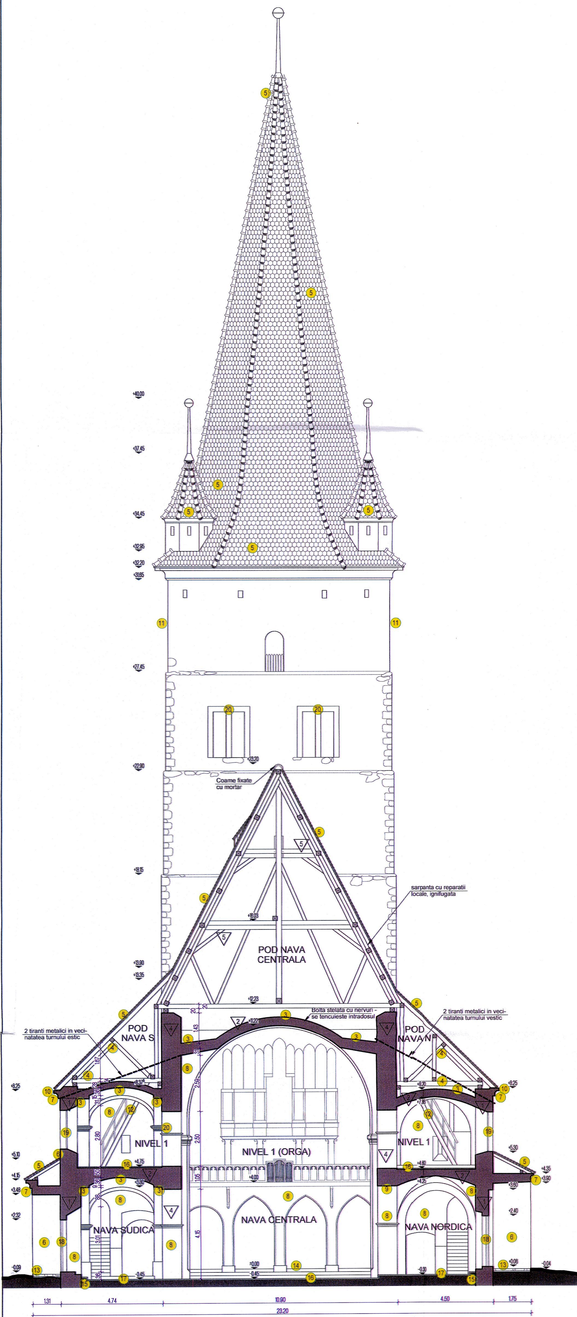
PROPUNERE BISERICA - SECTIUNE B-B scara 1:100
