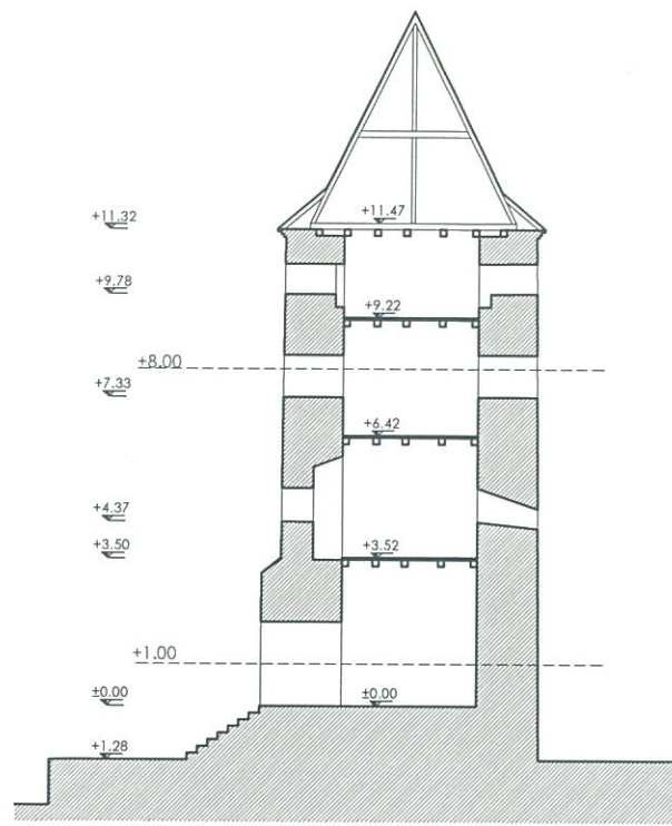
SECTIUNE
