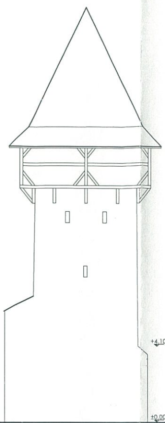
FATADA EST
