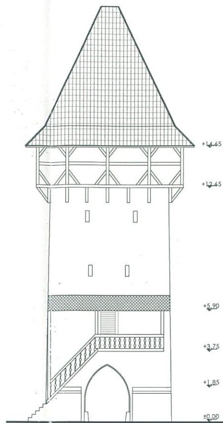
FATADA SUD
