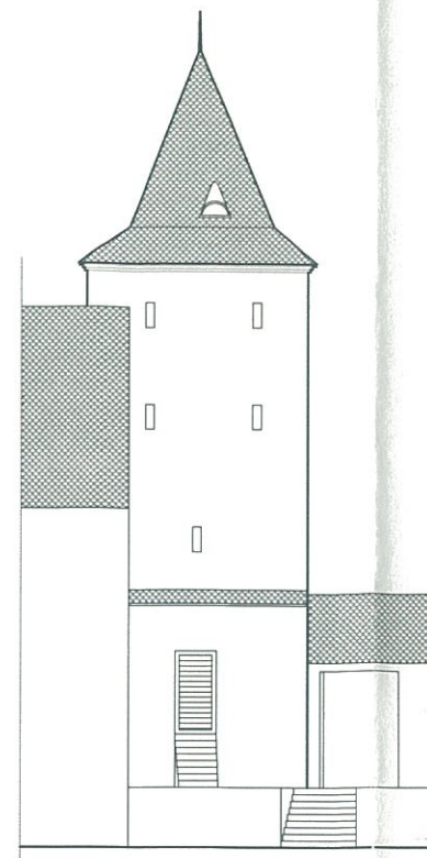
FATADA NORD
