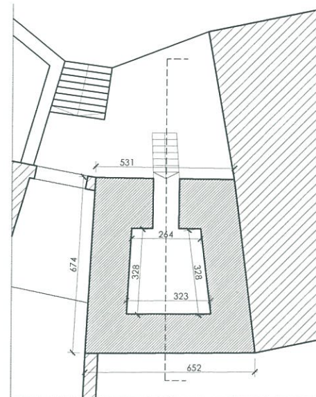
PLAN COTA +1.00m
