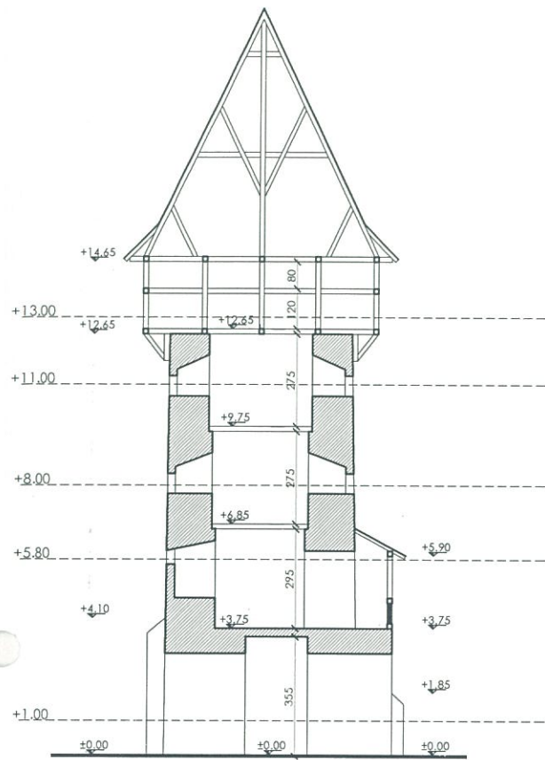
SECTIUNE TRANSVERSALA
