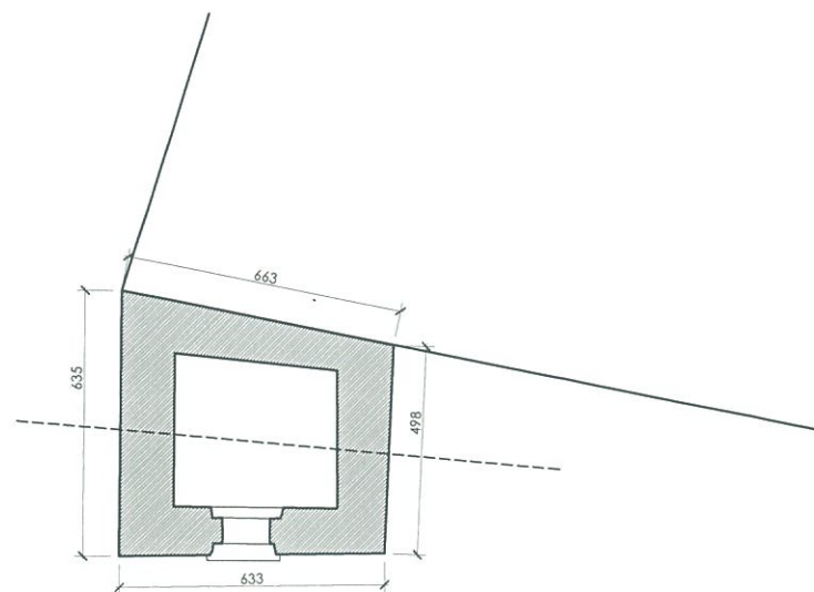
PLAN COTA +1.00m
