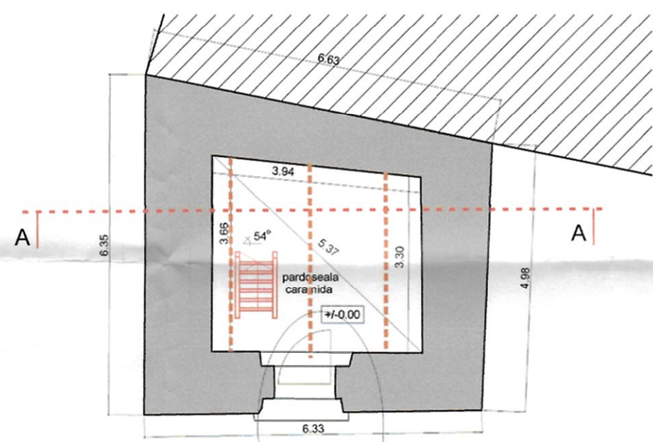
PLAN COTA +1.00 m
