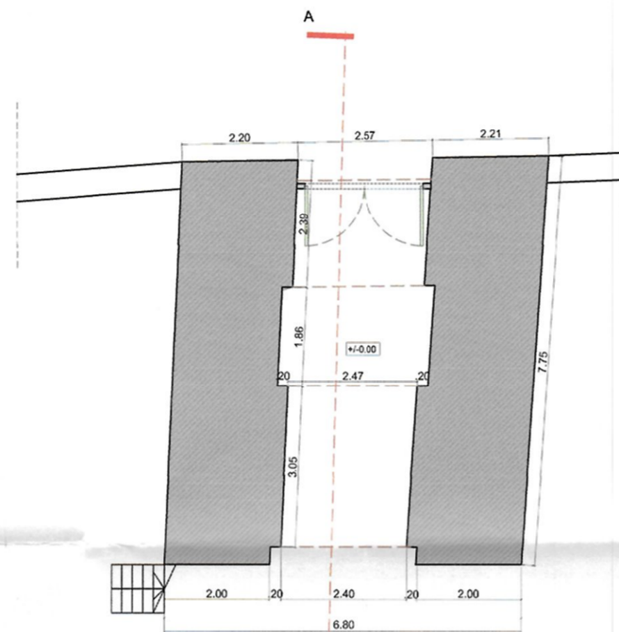
PLAN COTA +1.0 m
