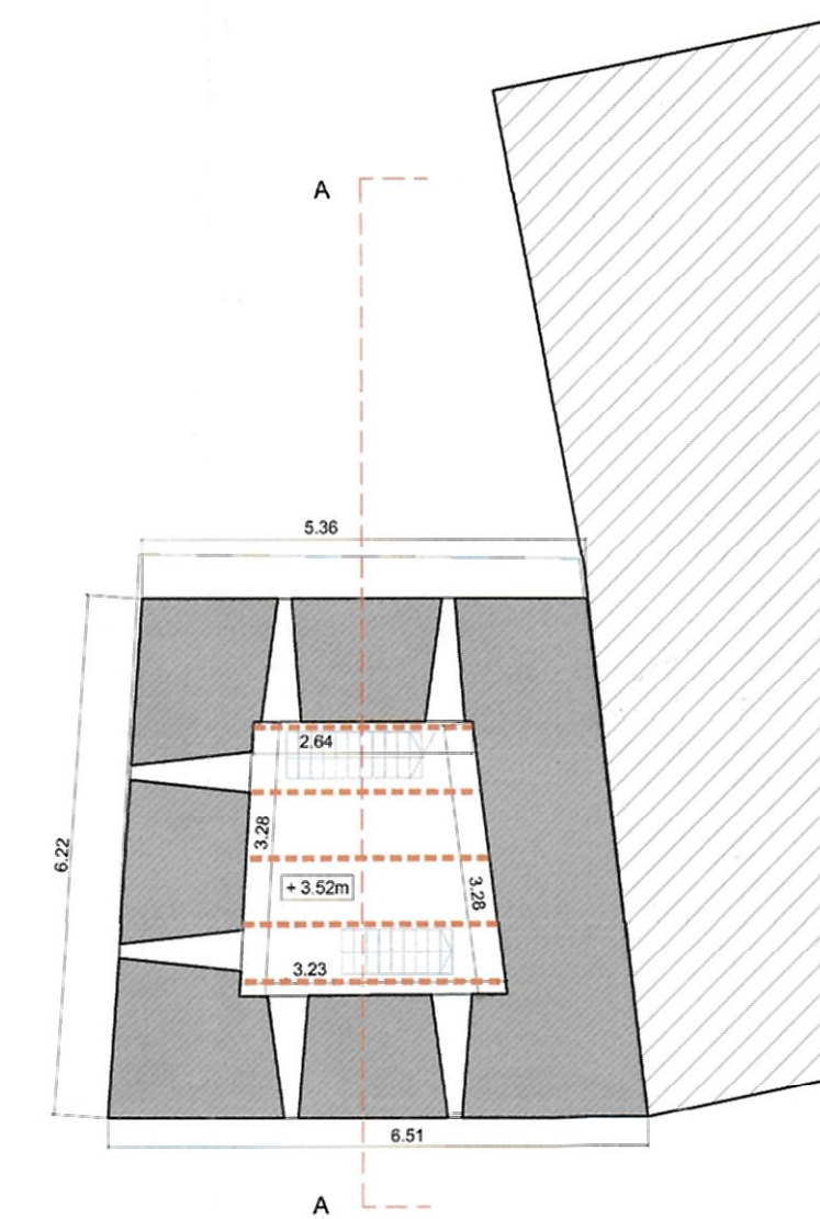
PLAN COTA + 4.65 M
