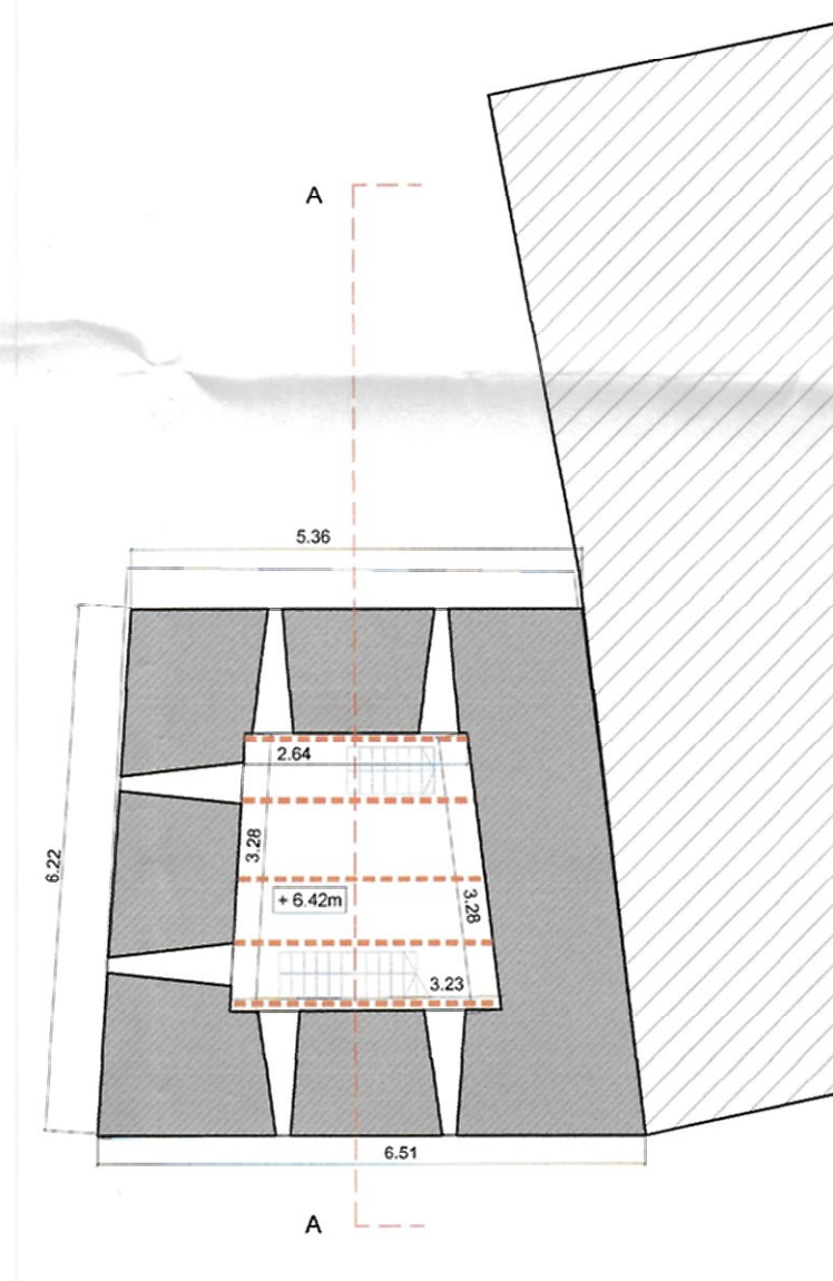
PLAN COTA +8.00m
