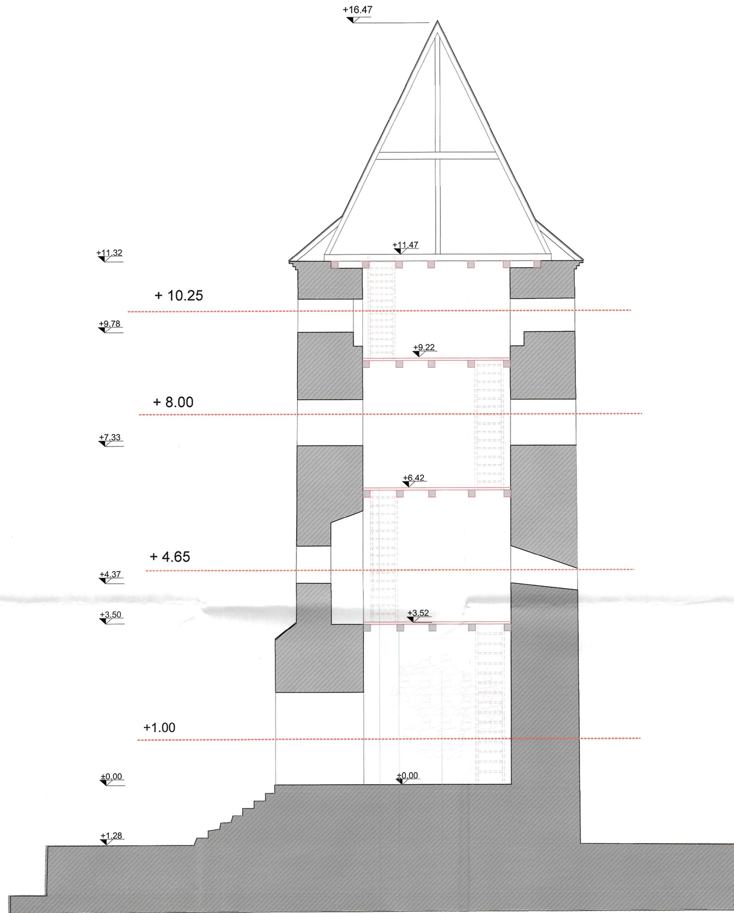
SECTIUNE A-A scara 1:50
