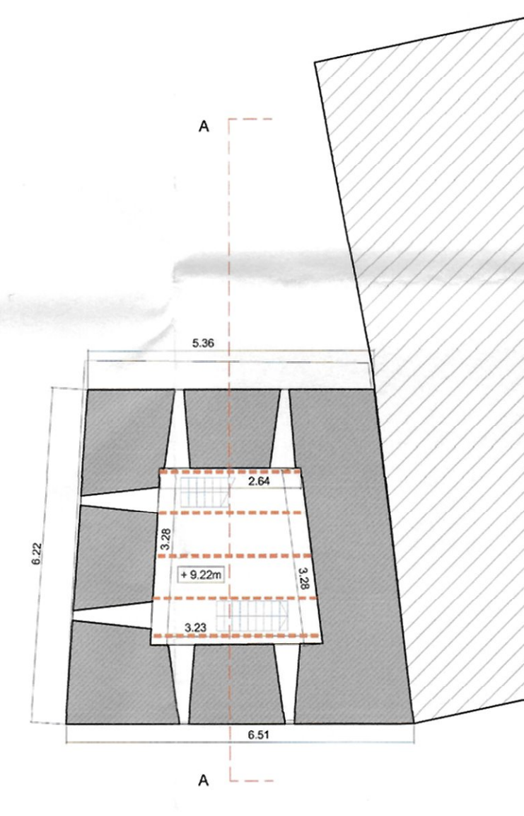
PLAN COTA + 10.25 m
